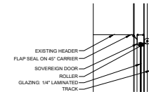
07 HEAD TYP SCALE: 1-1/2" = 1'
