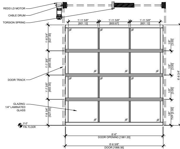
06 ELEVATION SCALE: 3/4" = 1'
