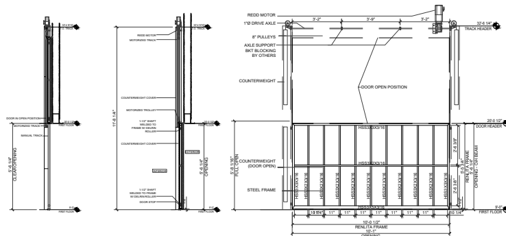
04 ELEVATION & SECTIONS MOTORIZED & NON SCALE: 3/8" = 1'
