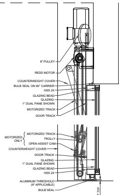
06 DOOR HEAD - SILL TYP SCALE: 1-1/2" = 1'
