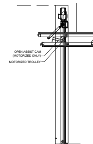
04 ELEVATION & SECTIONS MOTORIZED & NON SCALE: 1/2" = 1'
