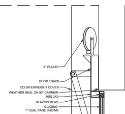
05 DOOR HEAD NON MOTORIZED SCALE: 1-1/2" = 1'
