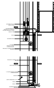
06 DOOR HEAD - SILL TYP SCALE: 1/2" = 1'
