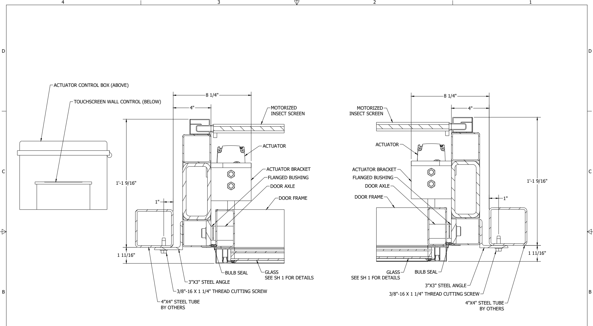
01 JAMB DETAIL
