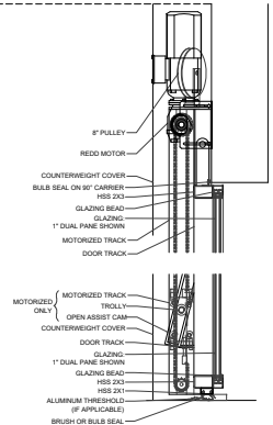
06 DOOR HEAD - SILL TYP SCALE: 1-1/2\"/>
