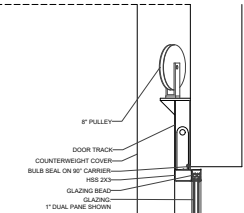
05 DOOR HEAD NON MOTORIZED SCALE: 1-1/2\"/>
