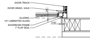
04 JAMB DETAIL SCALE: 1-1/2" = 1'
