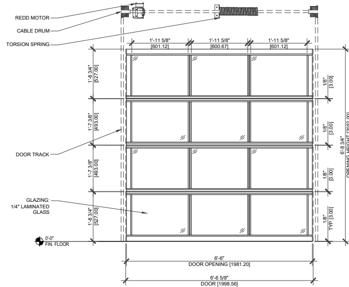
06 ELEVATION SCALE: 3/4" = 1'
