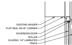
07 HEAD TYP SCALE: 1-1/2" = 1'
